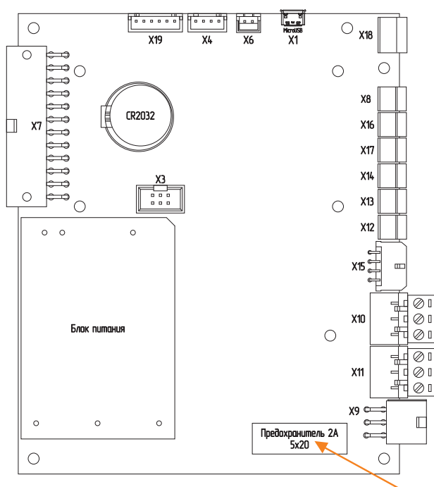
Рис.11 Плата контроллера
