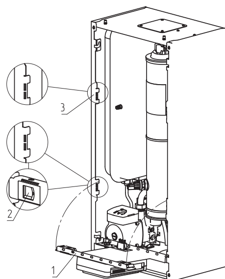
Рис.9 Откидывание кронштейна
