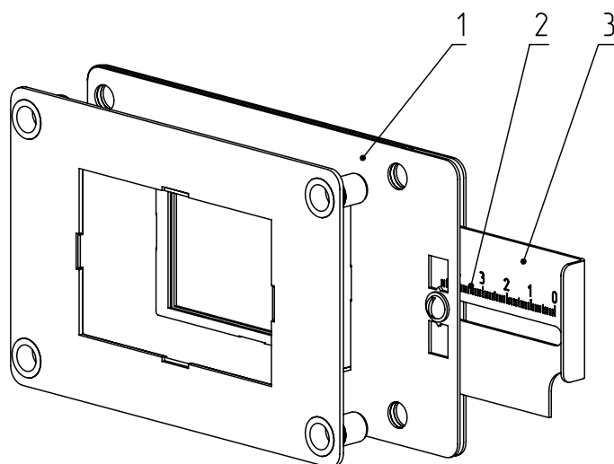
Рис.13 Заслонка вентилятора
