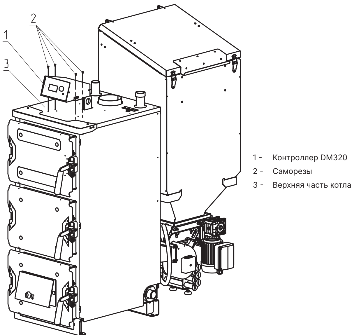
Рис.10 Монтаж контроллера
