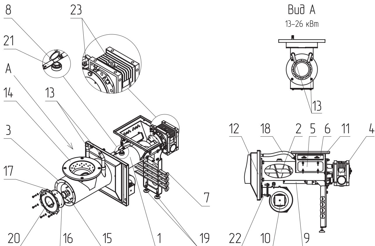
Рис.3 Механизм подачи топлива с горелкой котла
