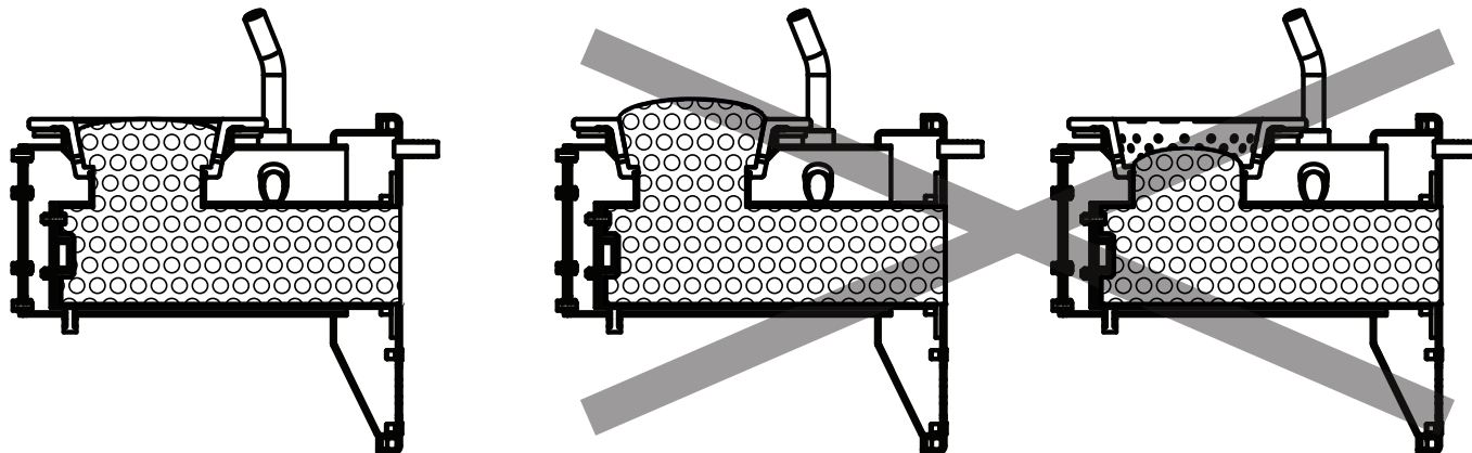
Рис.12 Настройка уровня топлива при горении
