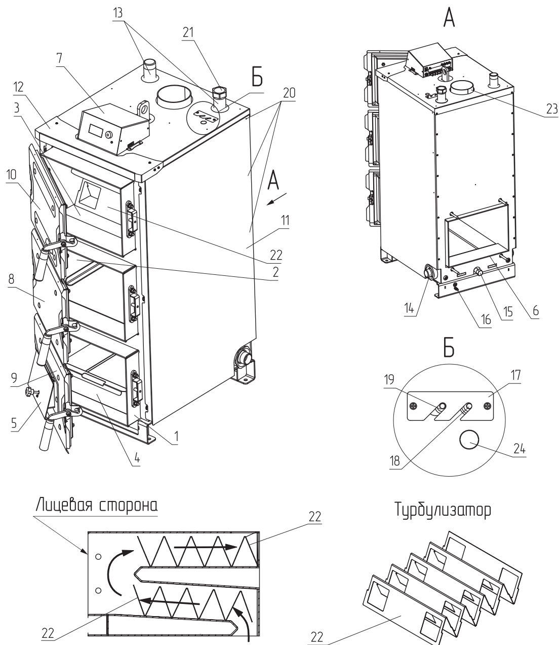
Рис.2 Конструкция теплообменника котла ZOTA «Rio»
