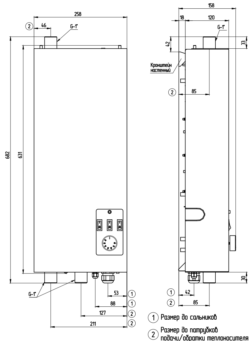
Рис.5 Габаритные размеры
